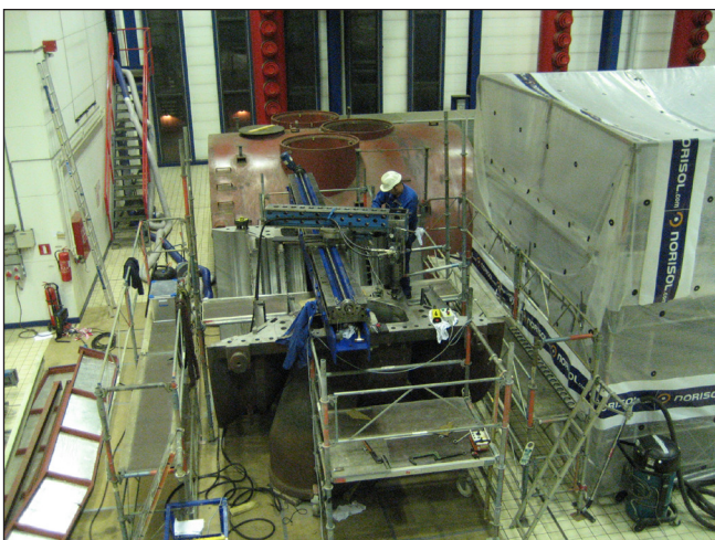
Mobil planfräsning av delningsplanet på nedre inre turbinhuset.
